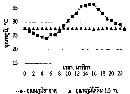
รูปที่ 11 อุณหภูมิใต้ดินสำหรับกลุ่มดินที่ 40 กลุ่มดินทราย
