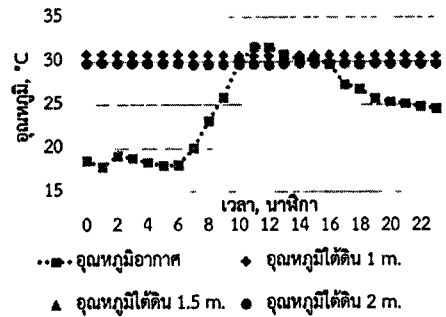
รูปที่ 9 อุณหภูมิใต้ดินสำหรับกลุ่มดินที่ 49 กลุ่มดินต้นถึงลูกรัง
