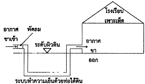
รูปที่ 7 การศึกษาสมรรถนะของระบบทำความเย็นด้วยท่อใต้ดิน
