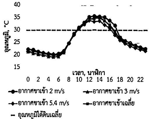
รูปที่ 13 อุณหภูมิอากาศเข้าของระบบทำความเย็นด้วยท่อใต้ดินที่ความเร็วลมต่างๆ และความเร็วลมเฉลี่ย
