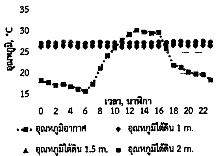
รูปที่ 10 อุณหภูมิใต้ดินสำหรับกลุ่มดินที่ 35 กลุ่มดินร่วนหยาบ
