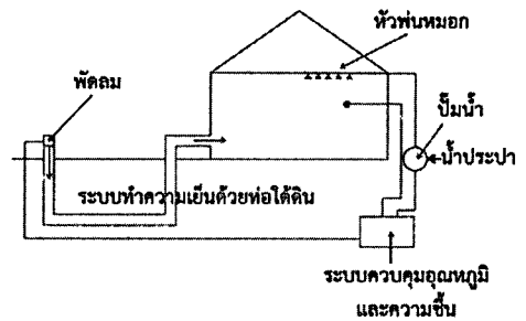
รูปที่ 8 การศึกษาสมรรถนะของระบบทำความเย็นด้วยท่อใต้ดินร่วมกับระบบพ่นหมอกอัตโนมัติ
