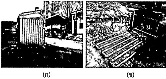
รูปที่ 12 โรงเรือนเพาะเห็ดและระบบทำความเย็นแบบท่อใต้ดินที่สร้างจริง
